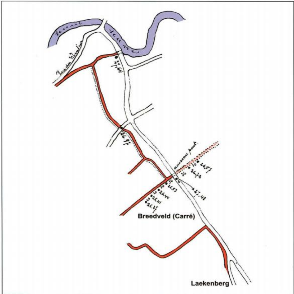
Plan opgesteld in 1924 naar aanleiding van het uitvoeren van verbeteringswerken ter voorkoming van overstromingen in de omgeving van het Breedveld. Uit de opmeting blijkt dat het Breedveld lager gelegen gebied is vergeleken met het niveau van de oevers van de Molenbeek ter hoogte van de monding in de Zenne. Dit verklaart waarom het Breedveld bij zware regelval vaak overstroomde.
